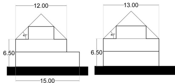
Schema bouwlagen/woonlagen - maximaal gabariet
